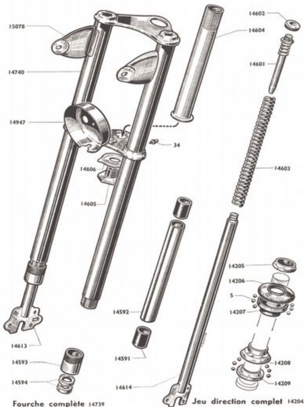
Fourche complète 14739
