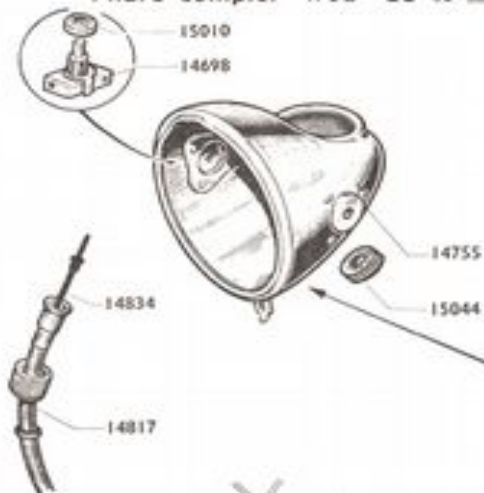
Phare complet trou de 60 14754
