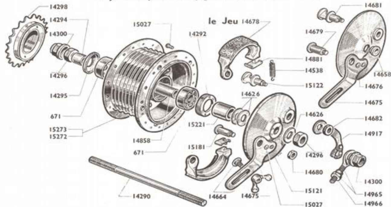
Moyeu complet avec pignon arrière 56 ds 14978
