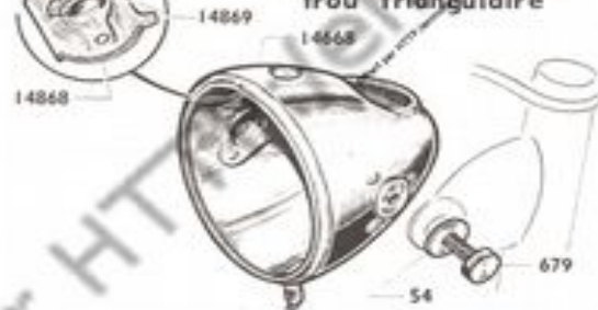
Phare complet LUXOR trou triangulaire 14467
