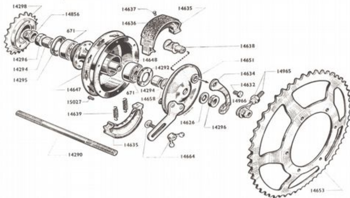
Moyeu complet avec pignon arrière 56 ds 14645
