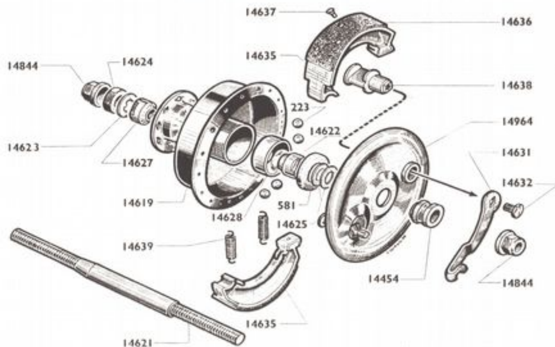
Moyeu avant complet 14618
