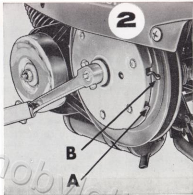
2. - Véhicule avec variateur.
